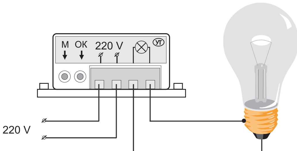
Схема подключения
