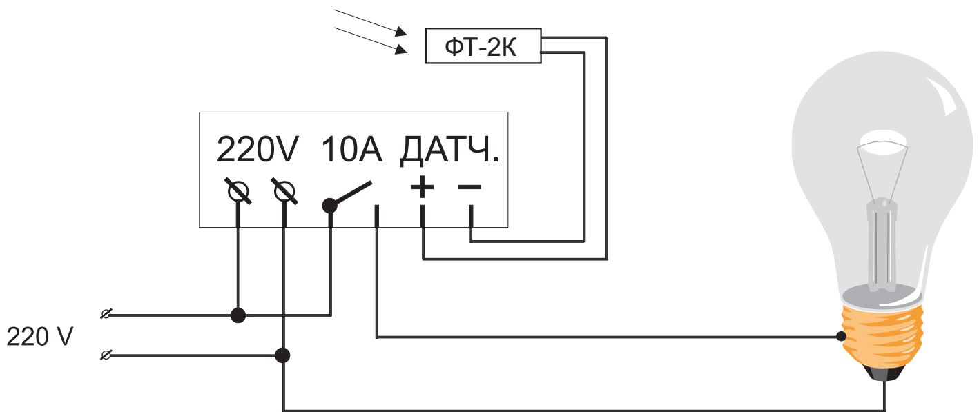
Схема подключения
