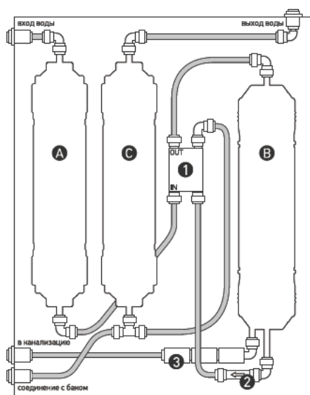
Рис. 2. Схема основного блока системы Expert Osmos.
